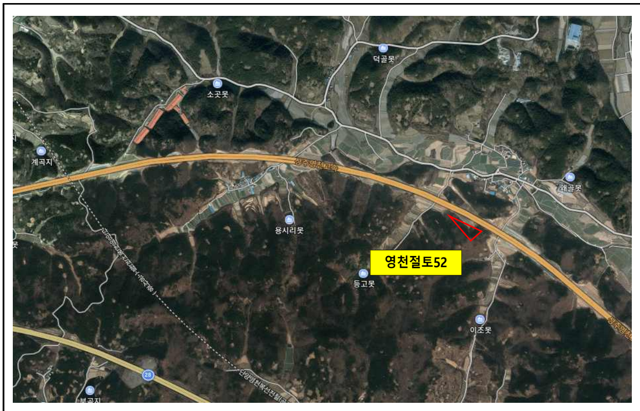
【그림 52-13】 영천절토52 검토대상 비탈면구간
