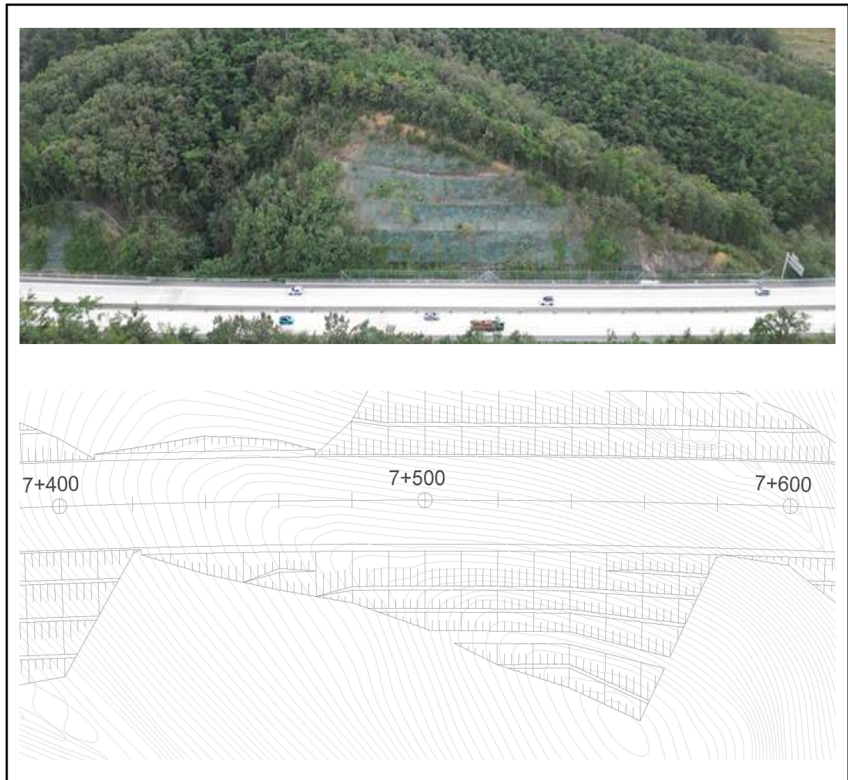
【그림 52-14】 영천절토52 검토대상 비탈면구간
