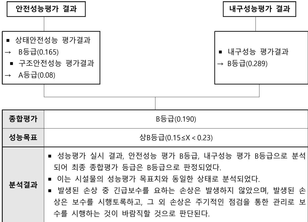
【표 52-90】 종합평가 결과 요약
