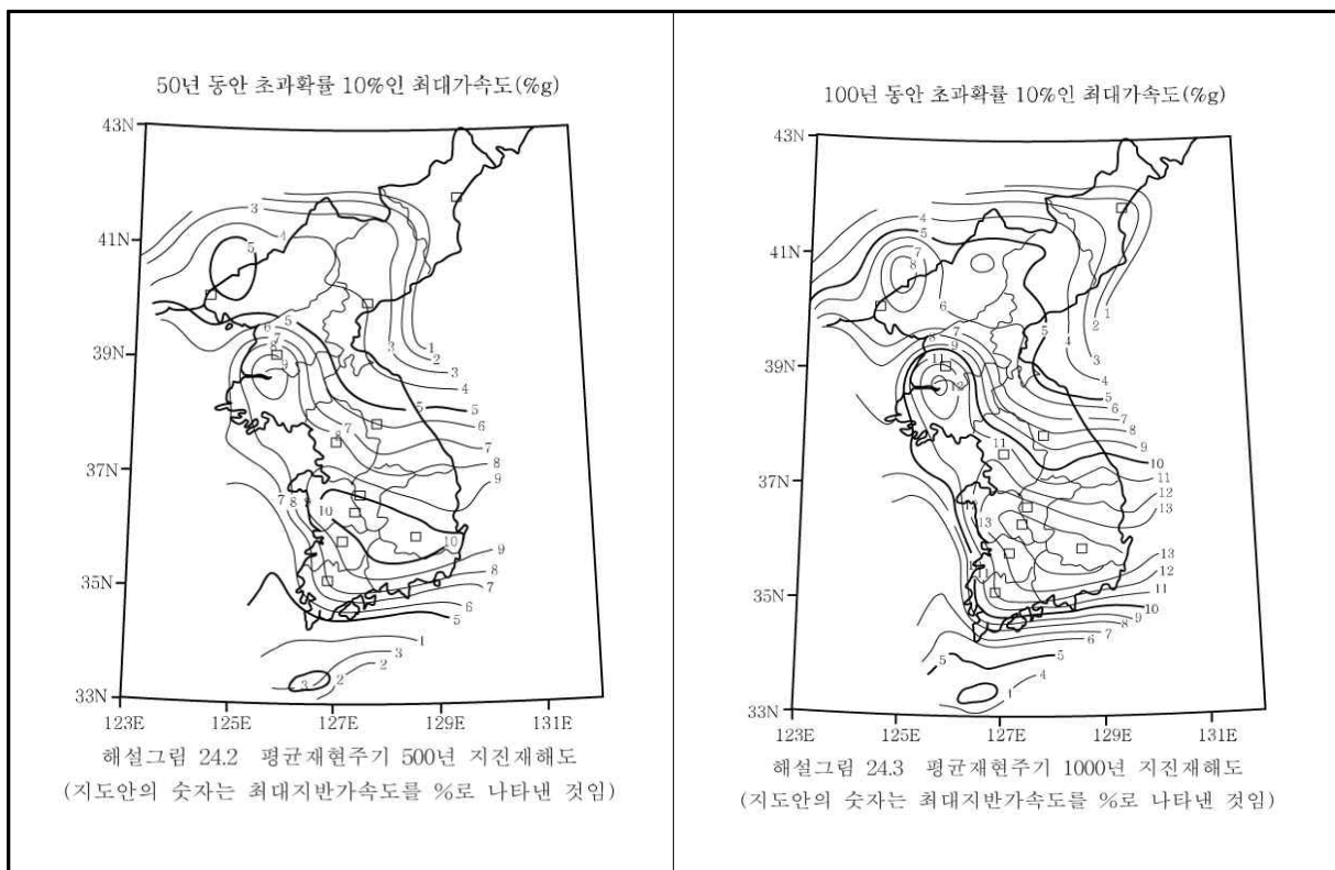
【그림 52-12】 평균재현주기 500년 및 1000년 지진재해도
