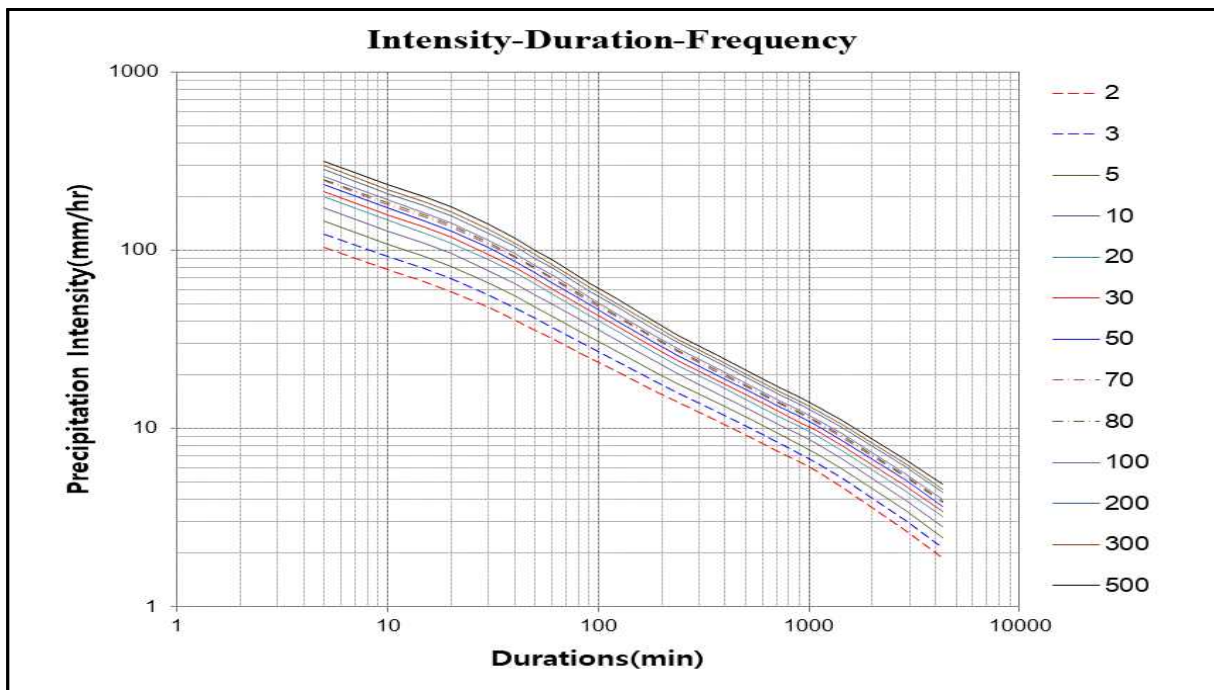
【그림 52-9】 영천지역 IDF곡선
